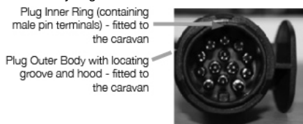
Fig.1 - 13 Pin Plug
